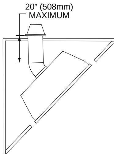
ÉVENTS RIGIDES
